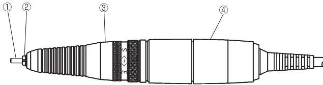
①ブランクバー ②コレットチャック ③セットリング ④モーターキャップ Blank Bur Collet Set Ring Motor Cap
